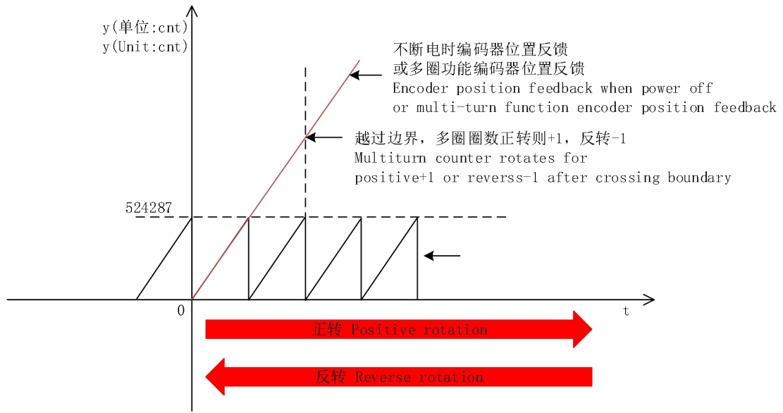
图 9-1 位置反馈
