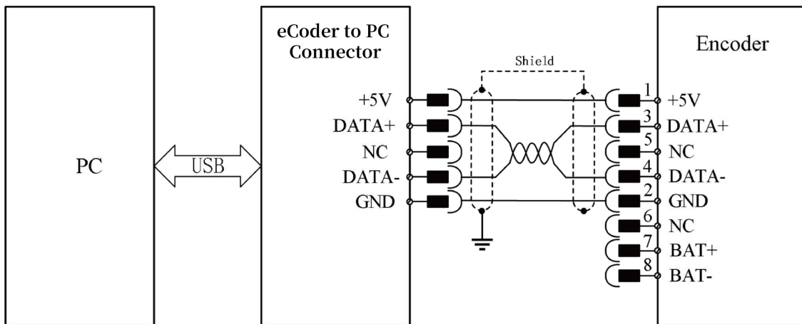
图 10-2 接线示例图
